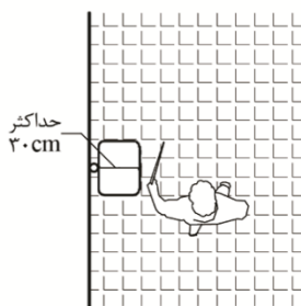
شکل شماره ۳۰: پیش‌آمدگی اشیای نصب‌شده روی پایه یا ستون
