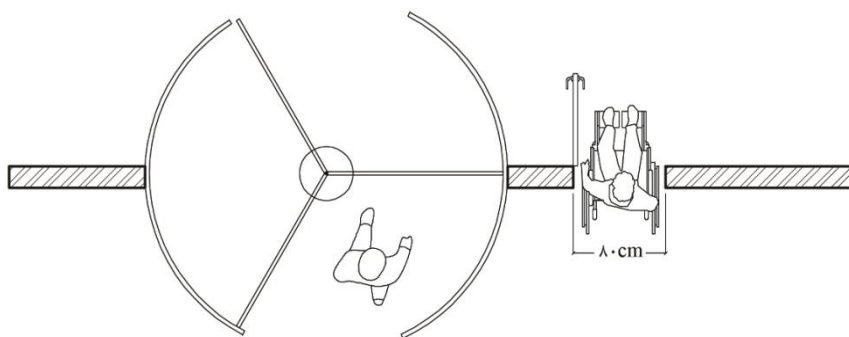
شکل شماره ۷۰: وجود یک لنگه در لولایی کنار در گردان
