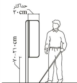
شکل شماره ۳۰: پیش‌آمدگی اشیای نصب‌شده روی پایه یا ستون
