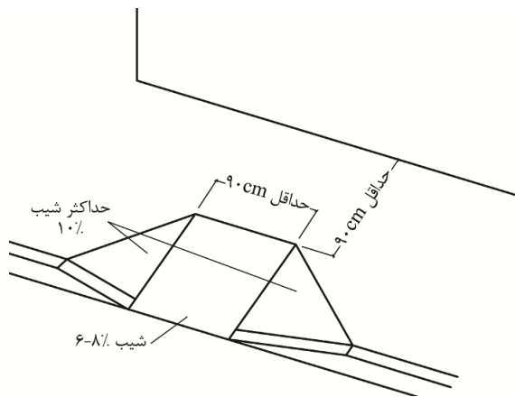
شکل شماره ۳۲: رمپ جدول
