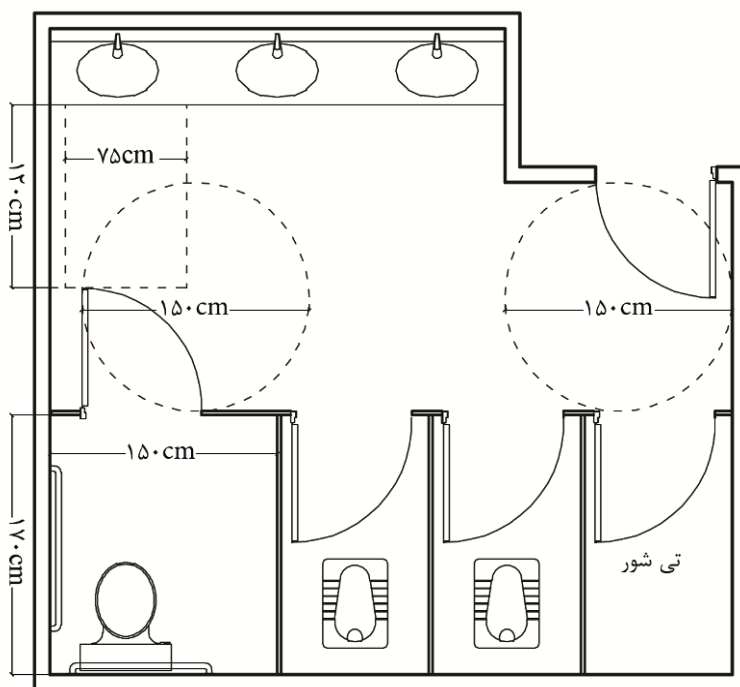
شکل شماره ۵۲: نمونه ابعاد سرویس بهداشتی عمومی برای دسترسی صندلی چرخدار
