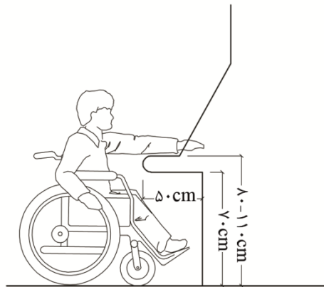
شکل شماره ۴۹: دستگاه خودپرداز دسترس‌پذیر
